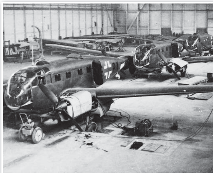
Montáž letadel Siebel Si 204D v pražském Aeru, stroj VE+PX v popředí nesl výrobní číslo 251203.
