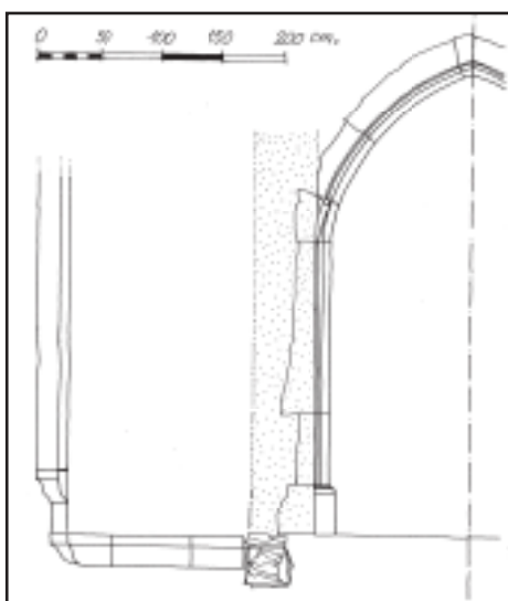
zaměření hradní kaple z parkánu (R. Vřla)
