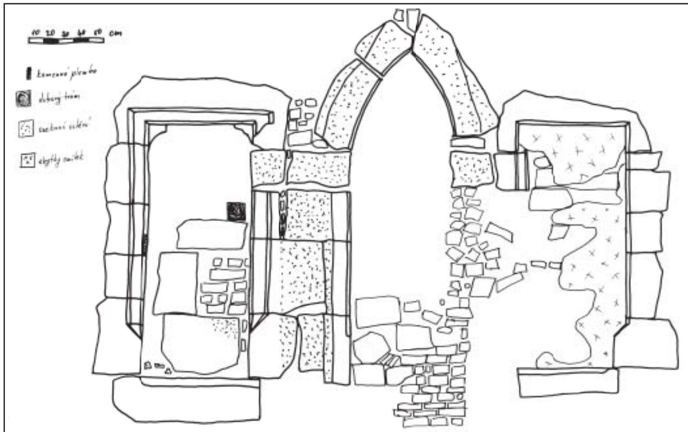
zaměření hradní kaple se dvěma vchody a nikou uprostřed z interiéru hradního paláce (P. Svoboda)
